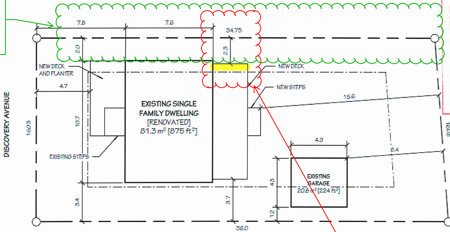
3 SITE PLAN 1:150
